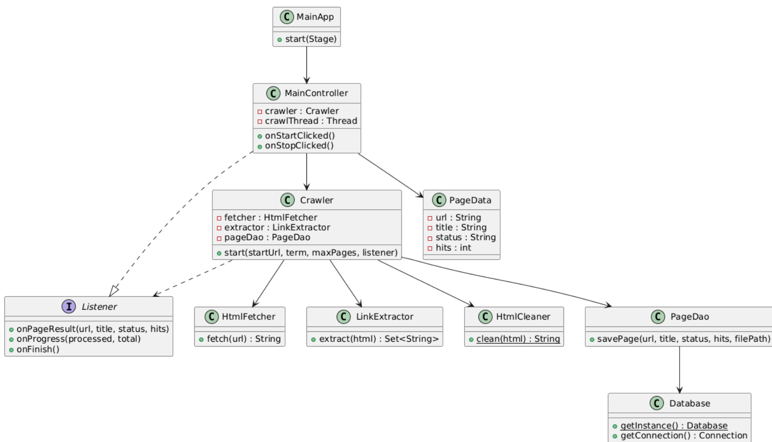
Діаграма класів системи «Web Crawler»
