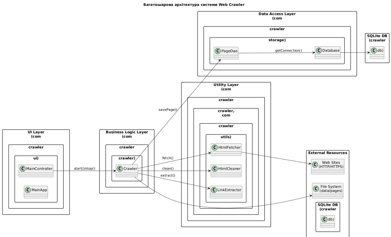
Рисунок 2.2.2.3 Діаграма патерну Layered Architecture
